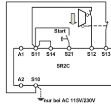
Fig. 4: Zweikanalige Schiebesechutzgitter-Überwachung mit Querschuss- und Masseschluss-Überwachung (Kategorie 4, bis PL e)
