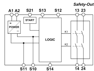
Abb. 1 Blockschaltbild SR2C
