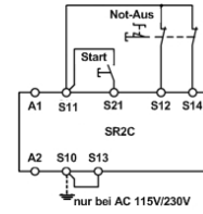
Fig. 2: Zweikanalige Not-Halt-Schaltung mit Masseschluss-Überwachung (Kategorie 3, bis PL d)
