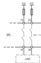
Fig. 11: Anschluss zu schaltender Lasten an Sicherheitsschalter. (Beispielhafte Kontaktkonfiguration. Je nach Gerätetyp abweichend. Schaltspannungen „+V“ entsprechend techn. Daten)
