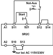
Fig. 3: Einkanalige Not-Halt-Schaltung mit Masseschluss-Überwachung (Kategorie 1, bis PL c)
