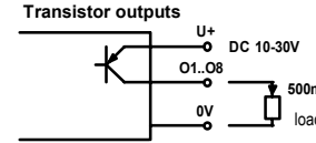
Fig. 4 Inputs / outputs
