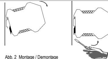
Abb. 2 Montage / Demontage
