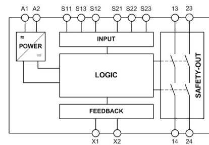
Abb. 1 Blockschaltbild S2HC
