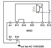
Abb. 6: Einkanalige Not-Halt-Schaltung mit Masseschluss-Überwachung (Kategorie 1, bis PL c / SIL 1)
