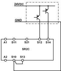
Abb. 8: Zweikanalige Not-Halt-Schaltung mit pnp-Halbleiterausgängen / OSSD-Ausgängen mit Querschusserkennung (Kategorie 4, bis PL e / SIL 3)
