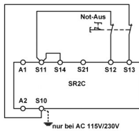
Abb. 4: Zweikanalige Not-Halt-Schaltung mit Querschuss- und Masseschluss-Überwachung (Kategorie 4, bis PL e / SIL 3)
