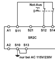
Abb. 4: Zweikanalige Not-Halt-Schaltung mit Querschuss- und Masseschluss-Überwachung (Kategorie 4, bis PL e / SIL 3)
