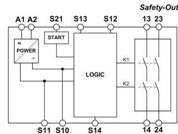
Abb. 1 Blockschaltbild SR2C
