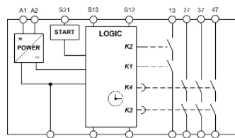
Abb. 1 Blockschaltbilder: SR4C (1unverz./3verz.);
